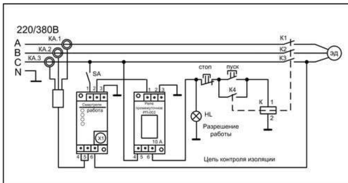
Схема подключения:
