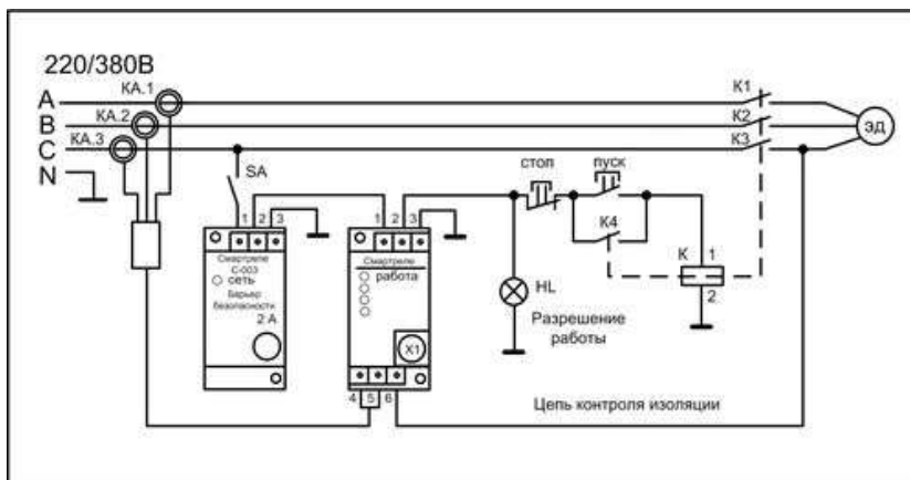
Схема подключения:
