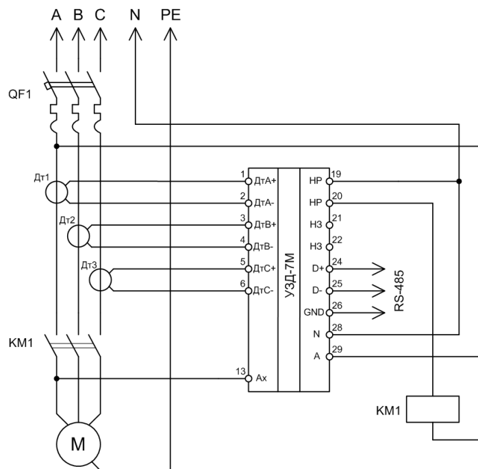
Рисунок 4 – Рекомендуемая схема включения: KM1 – магнитный пускатель; QF1 – автоматический выключатель; Дт1, Дт2, Дт3 – датчики тока.
