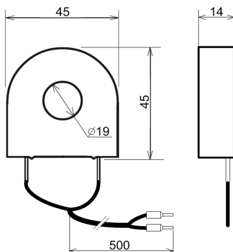
Рисунок 2.2 — Габариты датчиков тока для модификаций УЗД-7М 1,5-15А.
