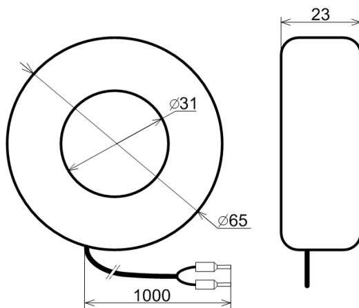
Рисунок 2.1 — Габариты датчиков тока для модификаций УЗД-7М 6,3-63А, 30-300А, 40-400А.
