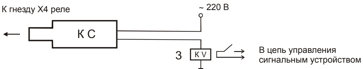
Рисунок 10 - внешний вид и варианты схем подключения контакта сигнального КС:
