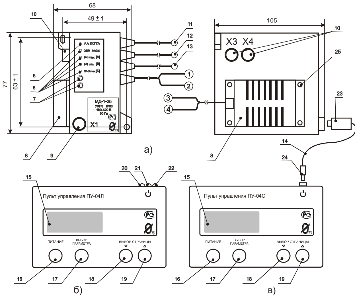
а) монитор двигателя МД-1 б) пульт управления ПУ-04Л (ПУ-04Т) в) пульт управления ПУ-04С
