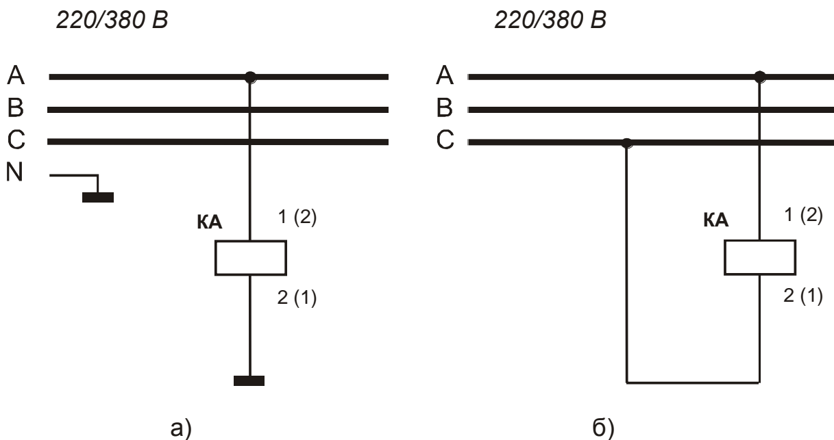
Рисунок 3 - схема питания монитора двигателя МД-1 от оперативного напряжения 220 В (а) или 380 В (б)
