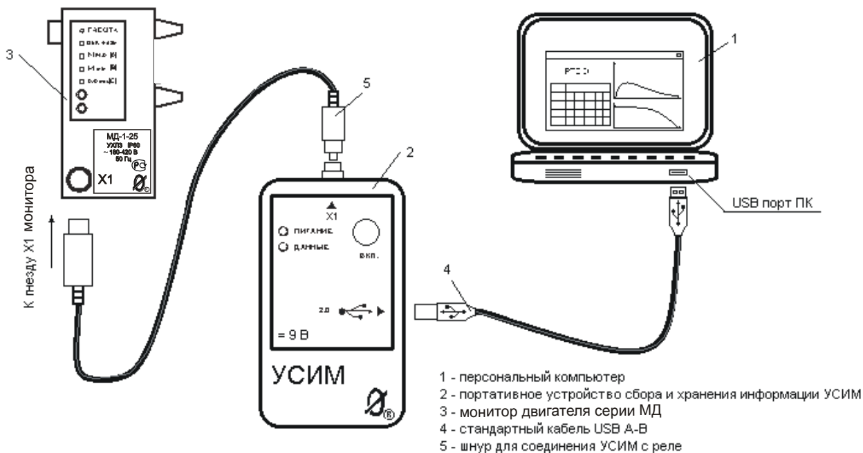
Рисунок 15 – подключение устройства сбора и хранения информации УСИМ к монитору двигателя серии МД и ПК.
