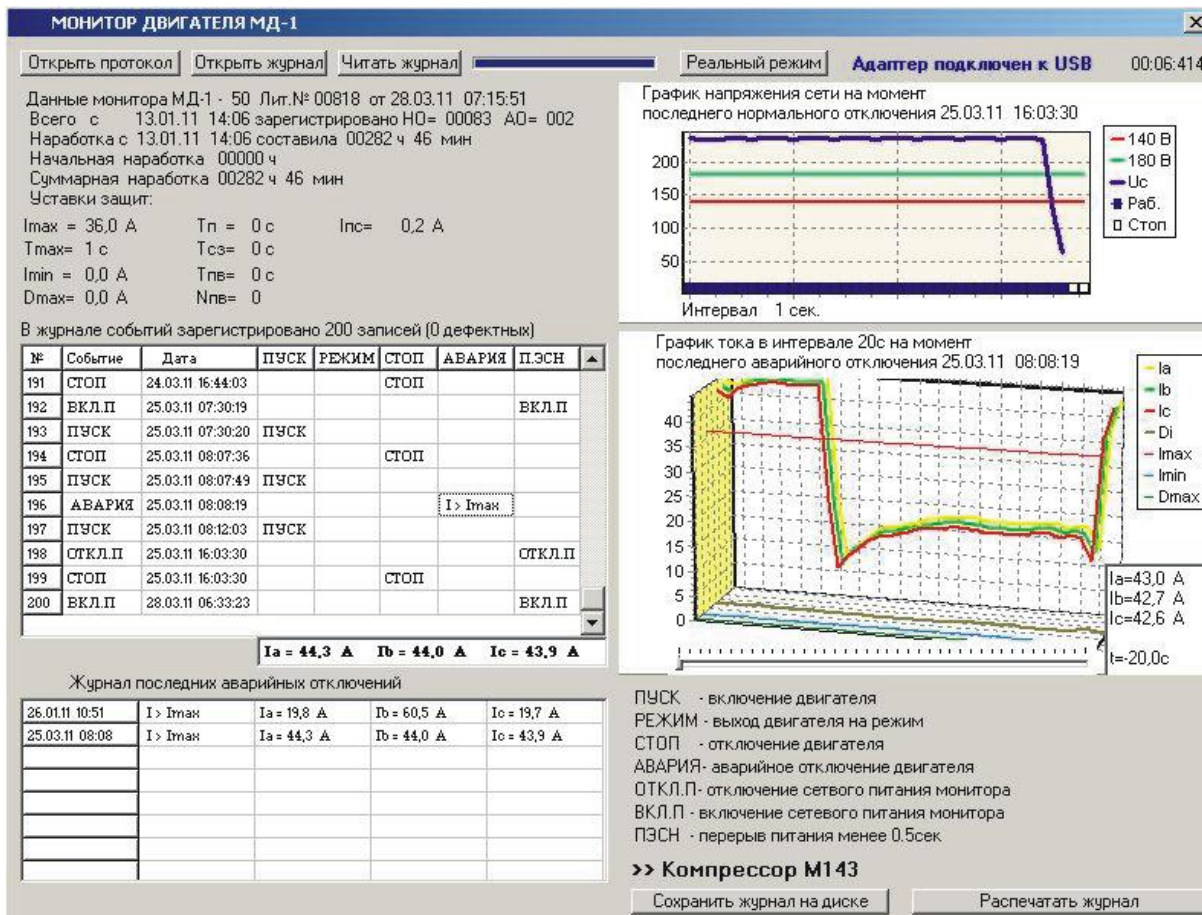
Рисунок 14 - отображение журнала событий монитора МД-1 на экране ПК.
