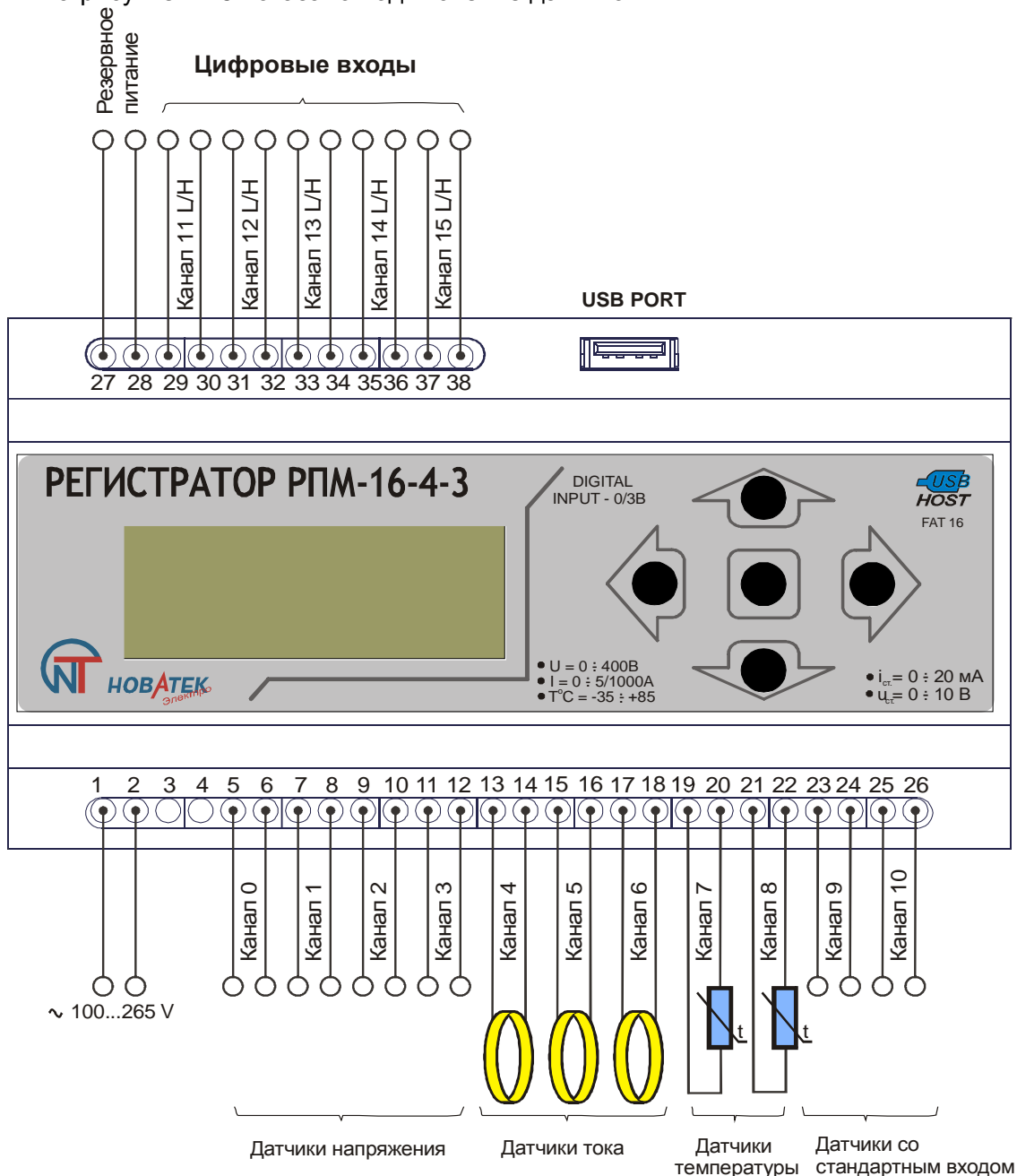
Рисунок 2.25 - Подключение датчиков
