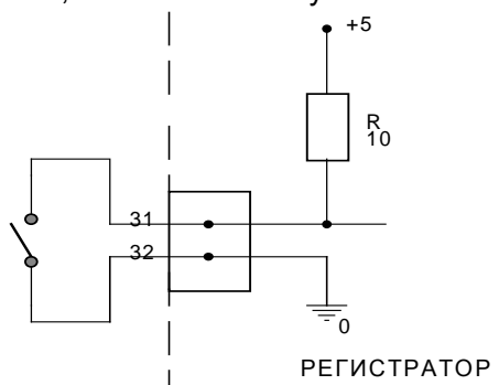
Рисунок 2.26 – Пример схемы подключения цифрового входа
