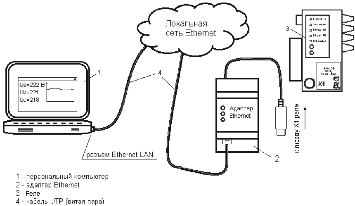
Рисунок 14 – включение реле РТЗЭ-В в локальную вычислительную сеть при помощи адаптера Ethernet
