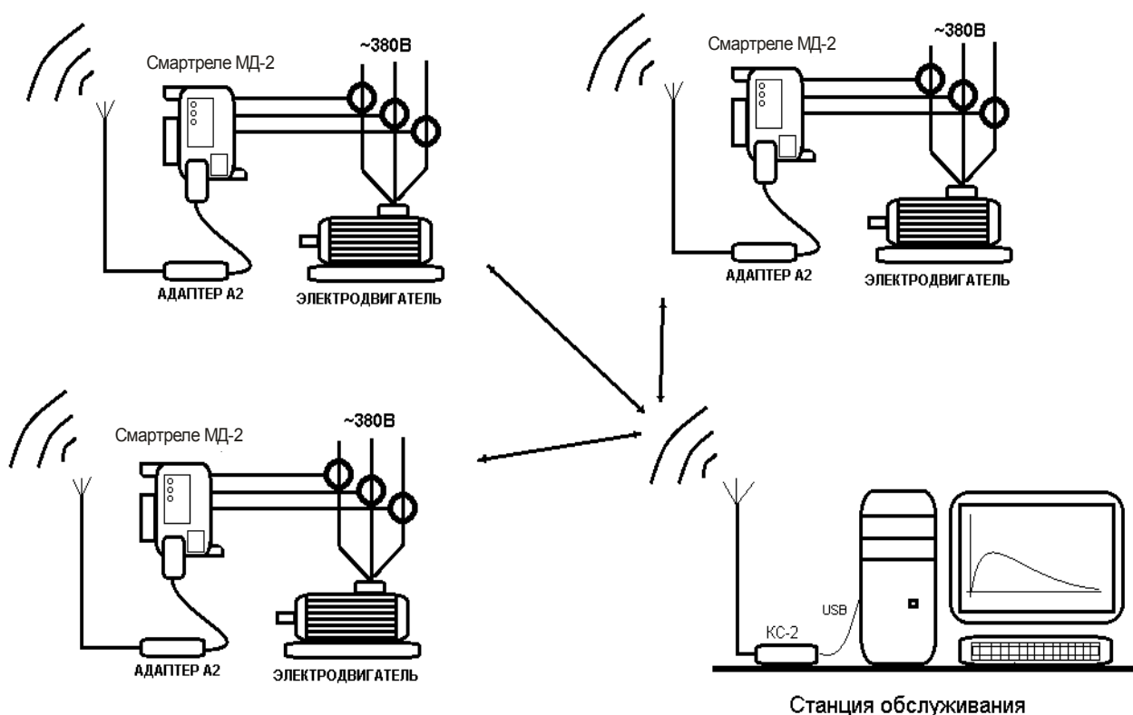
Рисунок 9 – схема организации связи в сети беспроводного доступа
