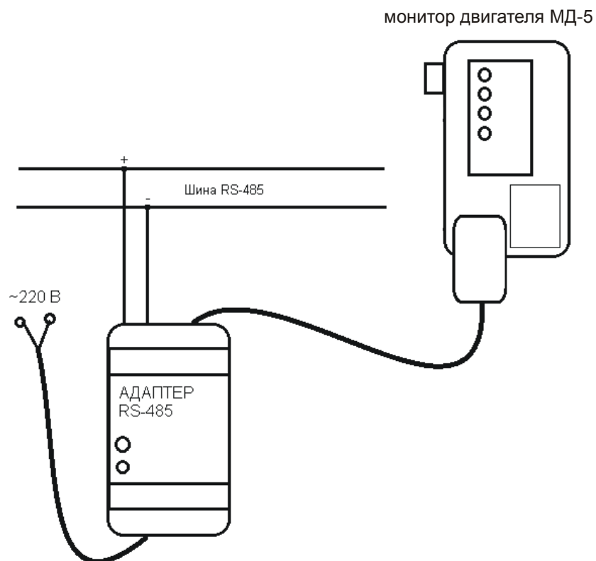
Рисунок 11 – подключение адаптера RS-485
