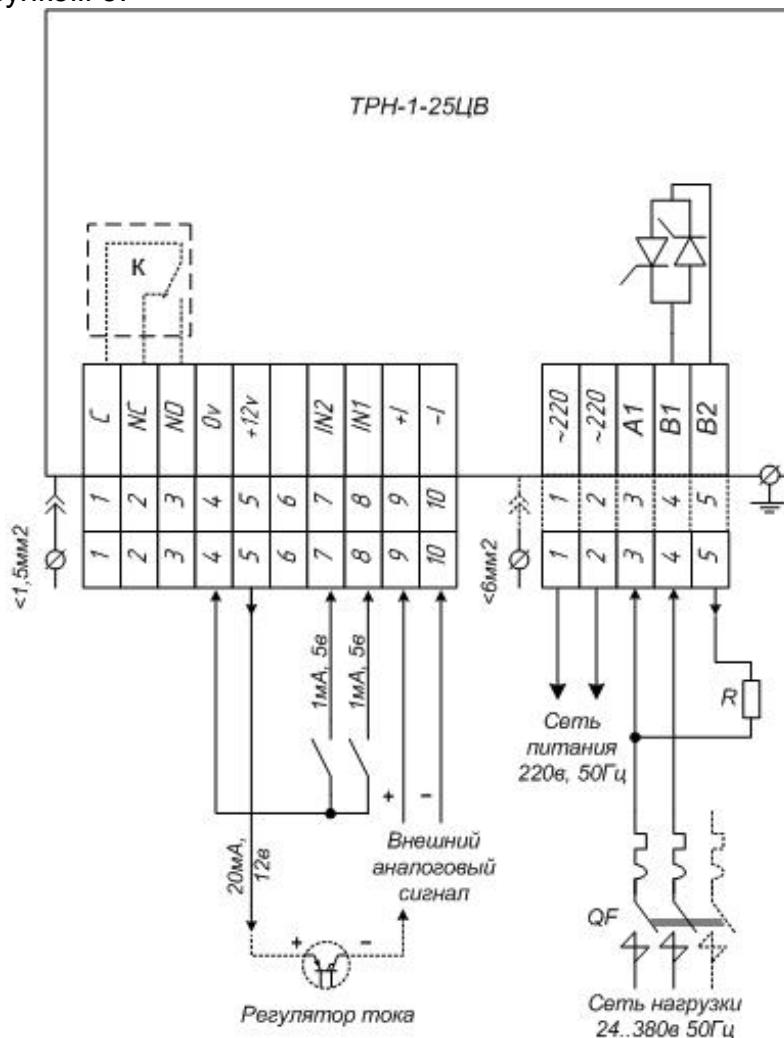
Рисунок 3. Схема подключения.
