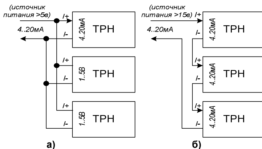
Рисунок 3. Схема подключения.
