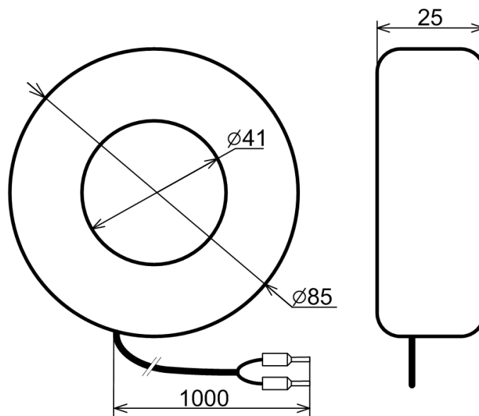
Рисунок 3 — Габариты датчиков тока ТТС 1528 для модификаций УЗД-11В 50-500А.
