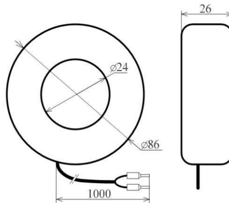
Рисунок 2 — Габариты датчиков тока Д-24 для модификаций УЗД-11В 1,0-10А и 8,4-84А.
