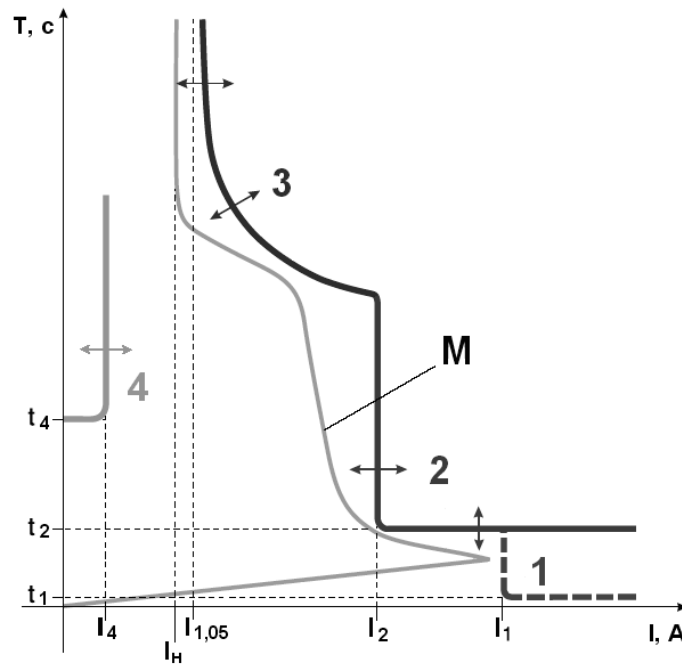
Рисунок 3 – Токовременная характеристика
