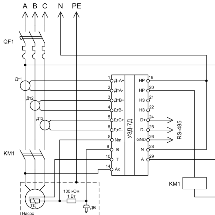
Рисунок 4 – Рекомендуемая схема включения: KM1 – магнитный пускатель; QF1 – автоматический выключатель; Дт1, Дт2, Дт3 – датчики тока; ТД – термодатчик; ДВ – датчик влажности.
